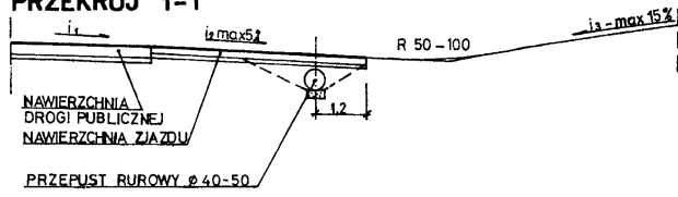
PRZEKRÓJ 1-1
