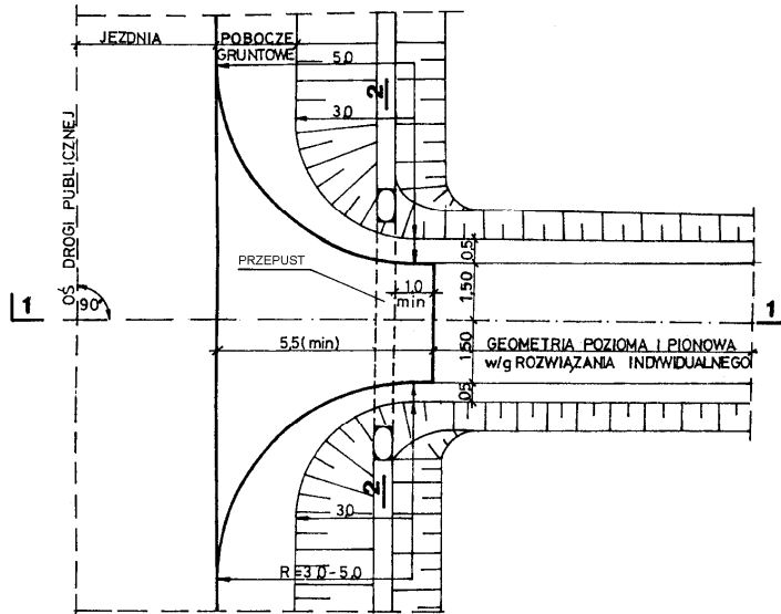
PRZEKRÓJ 1-1
