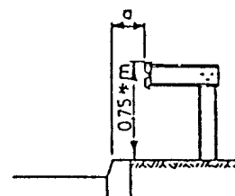
Załącznik 11.4. Profilowana taśma stalowa typu A i B, wg L. Mikołajków: Drogowe bariery ochronne, WKiŁ, 1983
