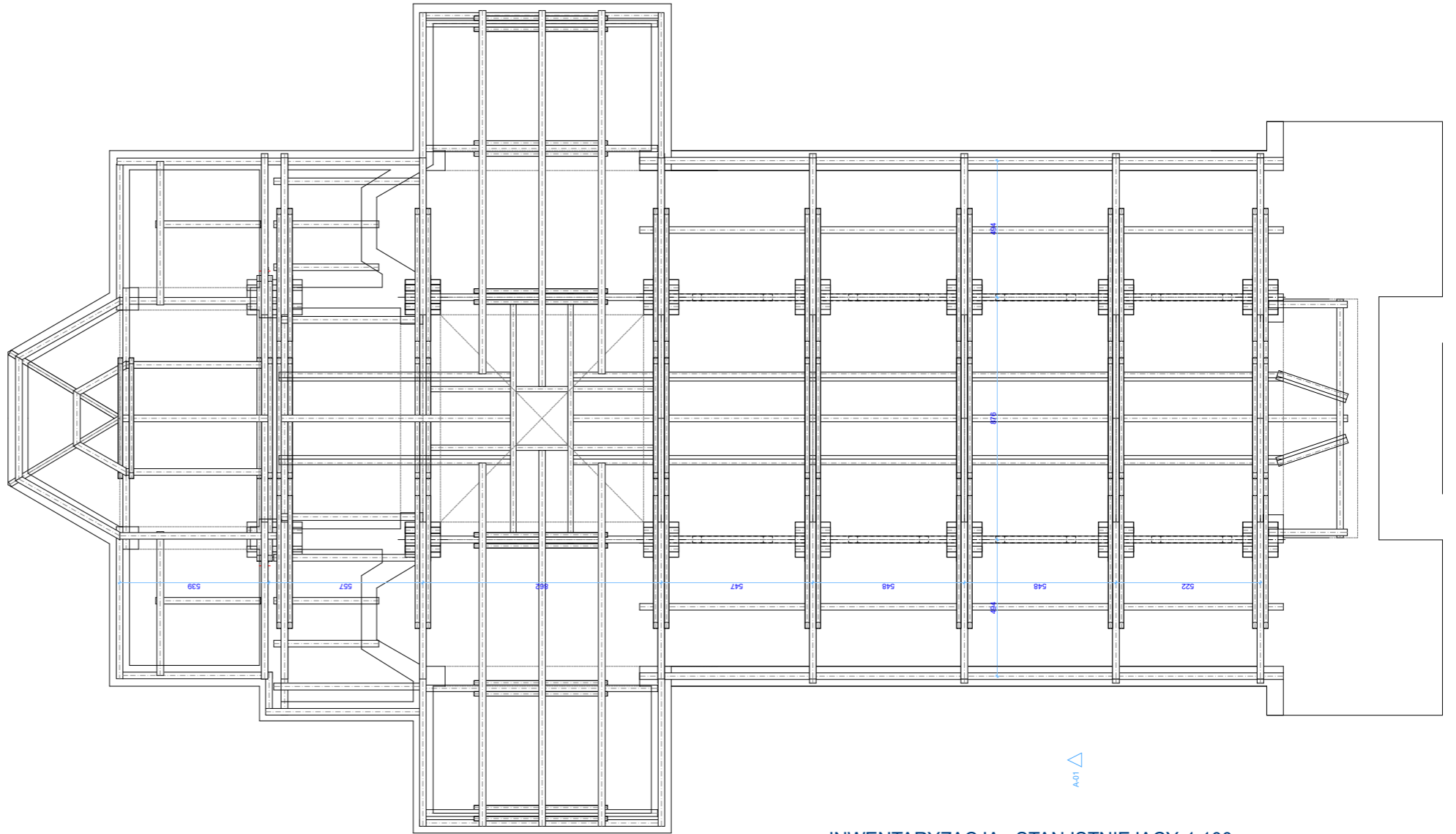
INWENTARYZACJA - STAN ISTNIEJĄCY 1:100
